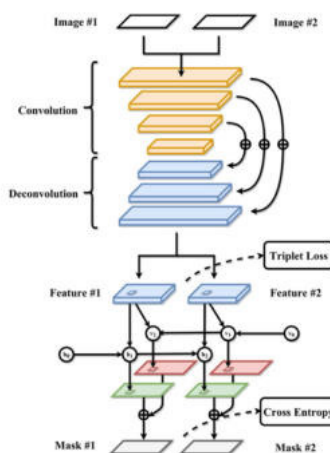
Figura 2.6: Arquitectura de la red neuronal presentada por Tang et al. (2018) . Esta arquitectura está compuesta por una CNN en la parte superior que extrae características de forma densa. Consta de una parte totalmente convolutiva para la representación de características a múltiples escalas y una parte de deconvolución para el refinamiento de detalles. La parte inferior es una estructura de red RNN bidireccional poco profunda para predecir la ubicación de los puntos clave en ambas imágenes.
