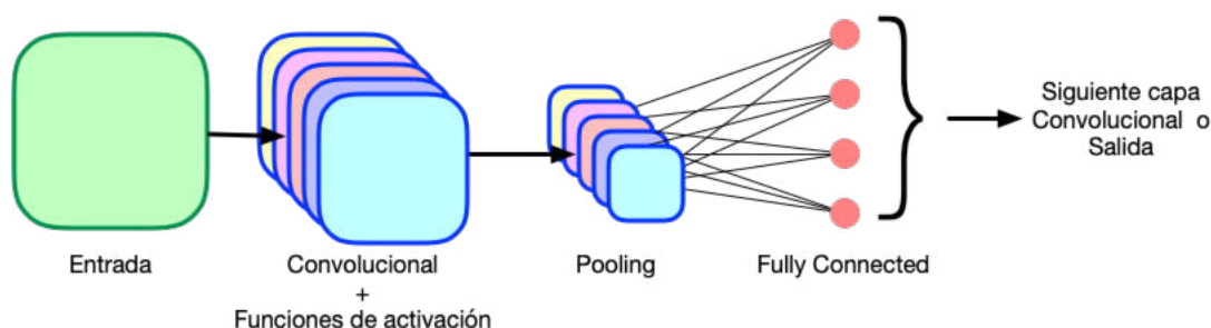
Figura 3.2: Arquitectura típica de una red CNN. Basado en el esquema que propone Amidi (2019) la arquitectura se compone de una capa de entrada, una capa de convolución, seguida de una capa de pooling y finalmente una capa totalmente conectada o la salida de la red.
